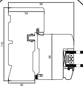
Seitenrahmen
