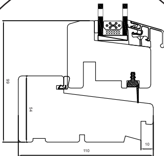
Untere Fensterrahmen
