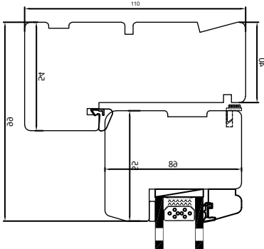
Oberer Fensterrahmen
