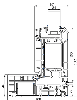
Bundkarm
