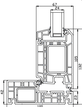
Bundkarm
