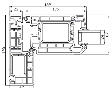
Sidekarm
