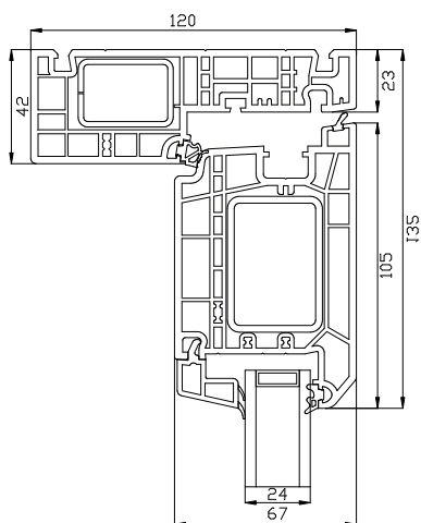
Overkarm
