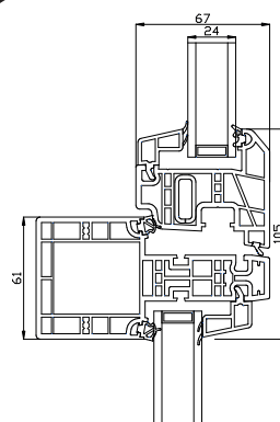
Tværpøst
