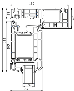
Overkarm
