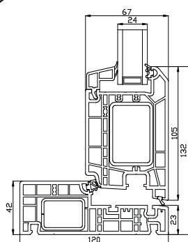
Onderdorpel
