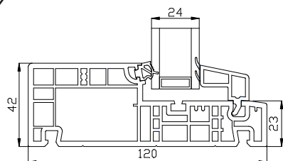
Onderdorpel
