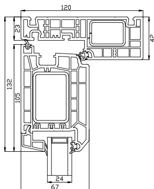
Bovendorpel
