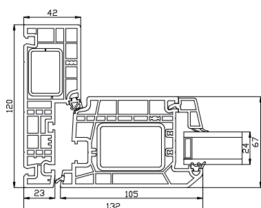
Zijstijl
