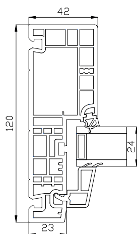
Zijstijl
