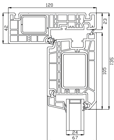
Bovendorpel
