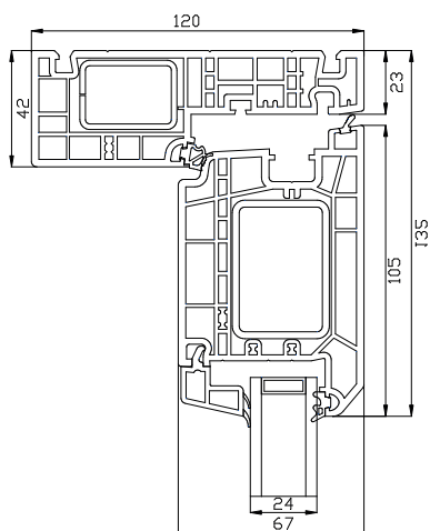
Bovendorpel
