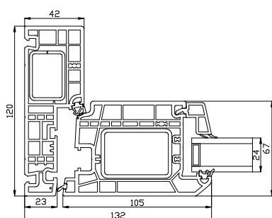
Zijstijl
