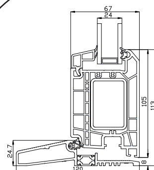
Aluminium onderdorpel
