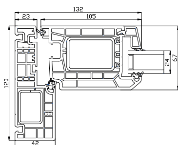
Zijstijl
