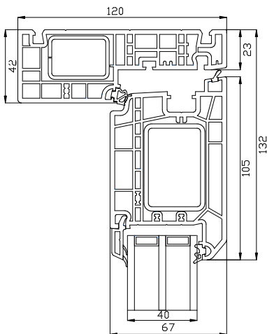
Bovendorpel
