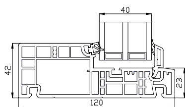
Onderdorpel
