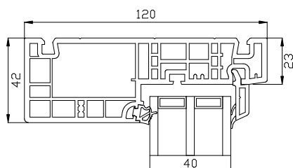
Bovendorpel
