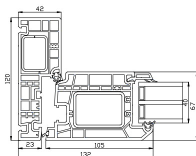
Zijstijl
