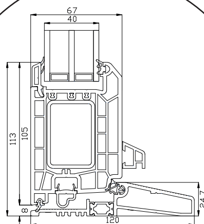
Onderdorpel
