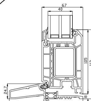
Aluminium onderdorpel
