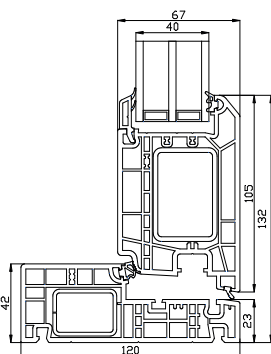
Onderdorpel
