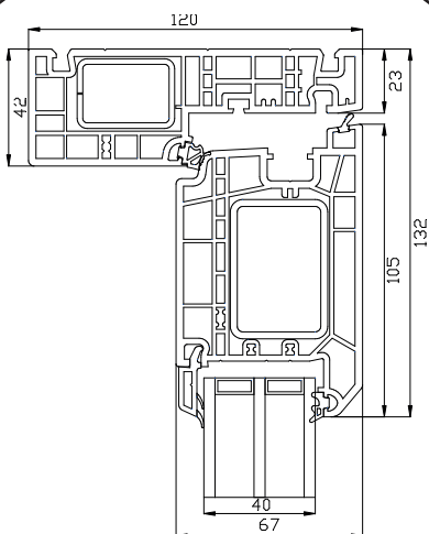
Bovendorpel
