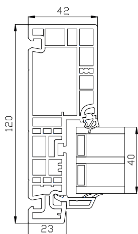
Zijstijl
