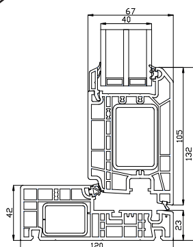
Onderdorpel
