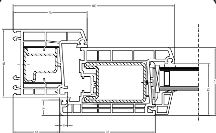
Zijstijl
