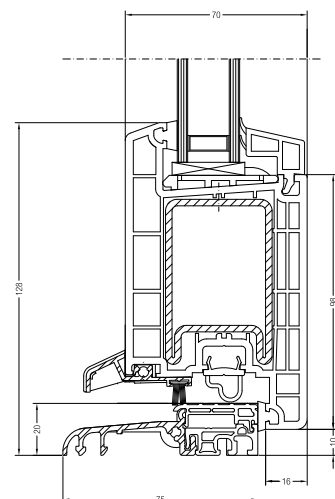
Onderdorpel
