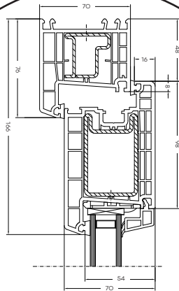
Bovendorpel
