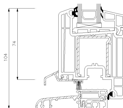
Onderdorpel
