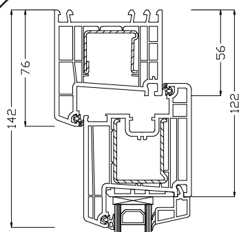
Bovendorpel
