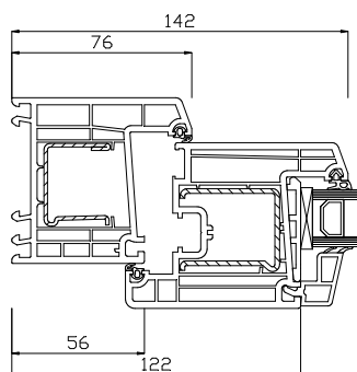
Zijstijl
