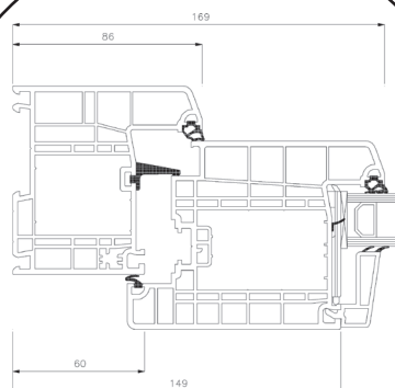
Zijstijl
