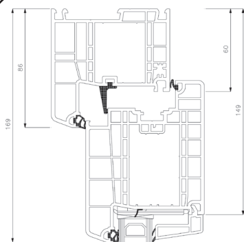
Bovendorpel
