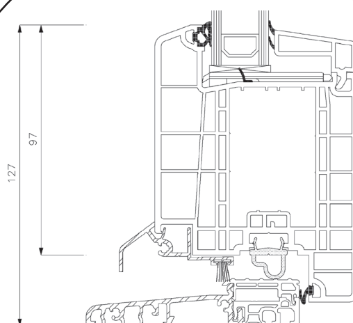
Onderdorpel
