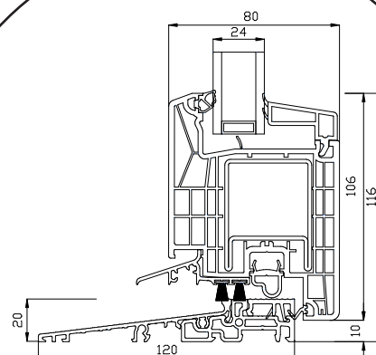
Aluminium onderdorpel
