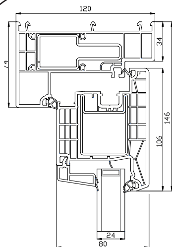
Bovendorpel
