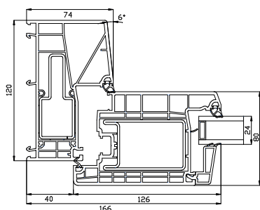
Zijstijl
