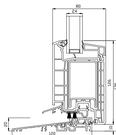
Onderdorpel
