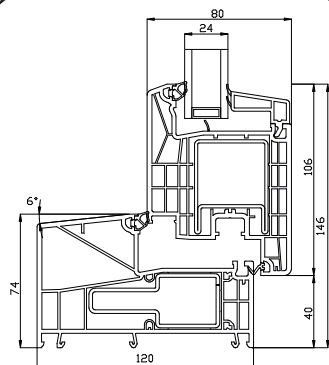
Kunststof onderdorpel
