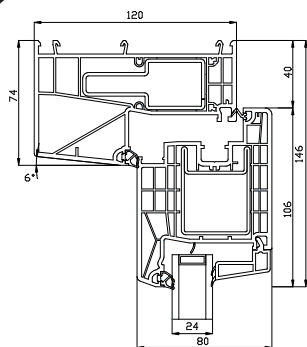
Bovendorpel
