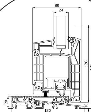
Aluminium onderdorpel
