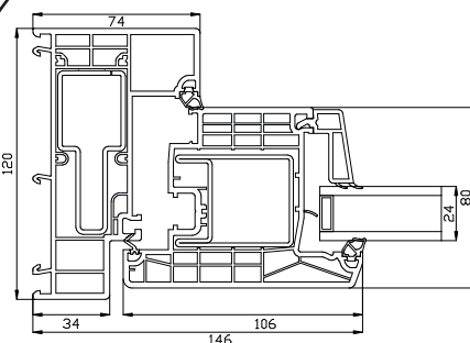
Zijstijl
