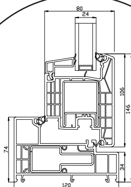
Kunststof onderdorpel
