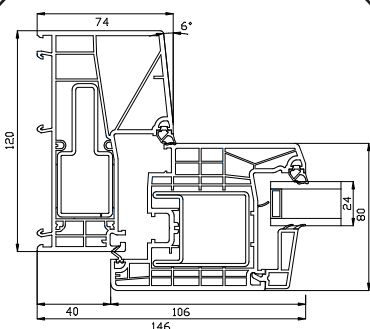
Zijstijl
