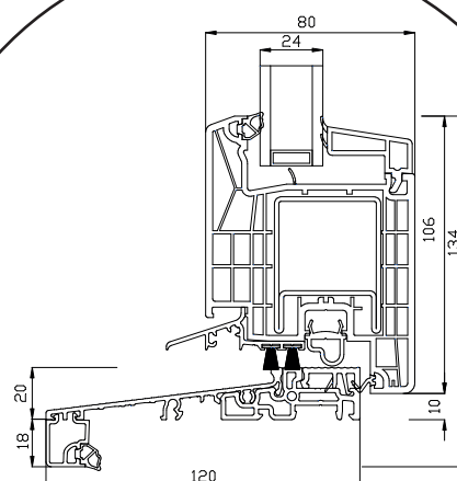
Aluminium onderdorpel
