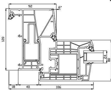
Zijstijl
