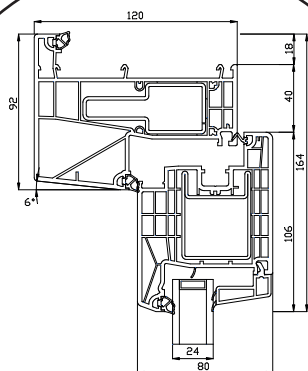
Bovendorpel
