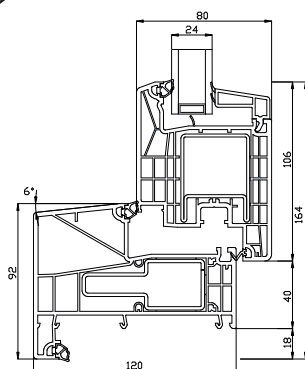
Kunststof onderdorpel
