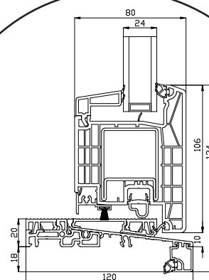
Aluminium onderdorpel
