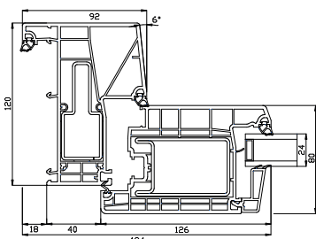
Zijstijl
