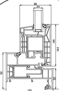
Kunststof onderdorpel
