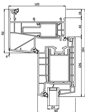
Bovendorpel
