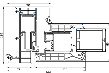
Zijstijl
