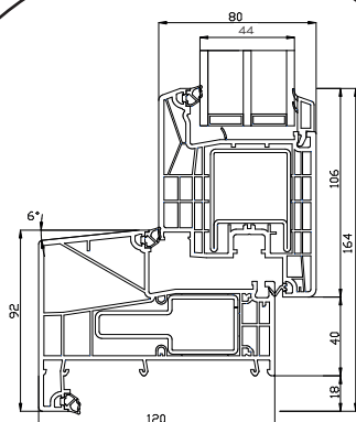
Kunststof onderdorpel
