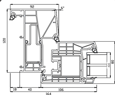
Zijstijl
