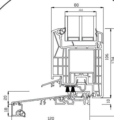
Aluminium onderdorpel
