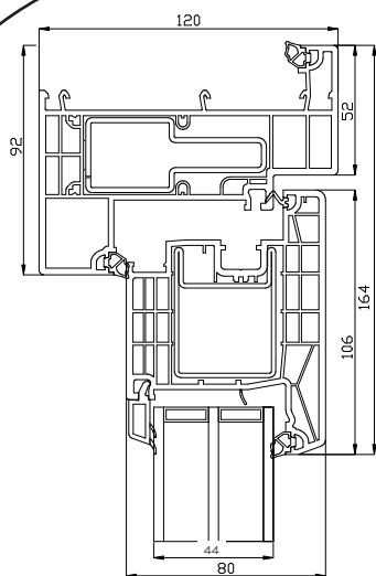
Bovendorpel
