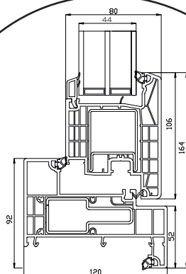
Kunststof onderdorpel
