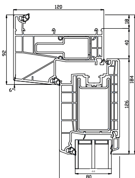
Bovendorpel
