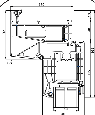
Bovendorpel
