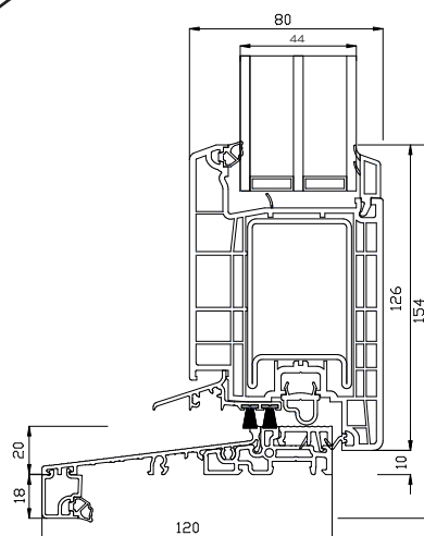
Onderdorpel
