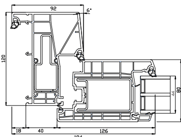
Zijstijl
