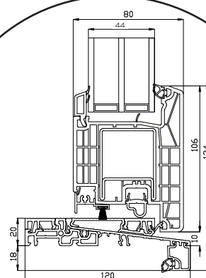
Aluminium onderdorpel
