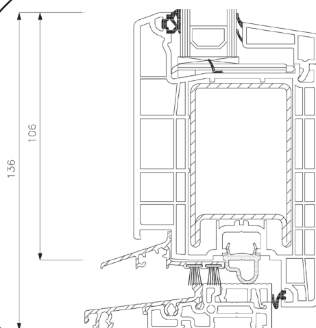
Onderdorpel
