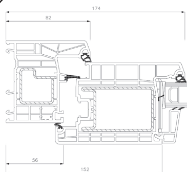
Zijstijl
