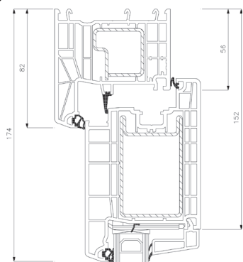
Bovendorpel
