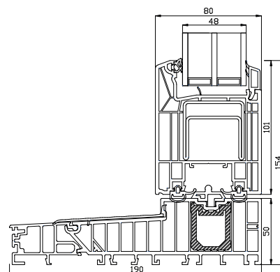
Onderdorpel
