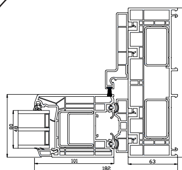
Zijstijl
