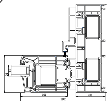
Zijstijl
