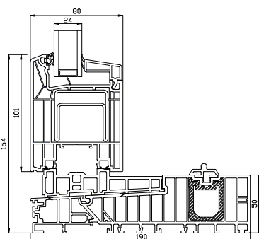
Onderdorpel
