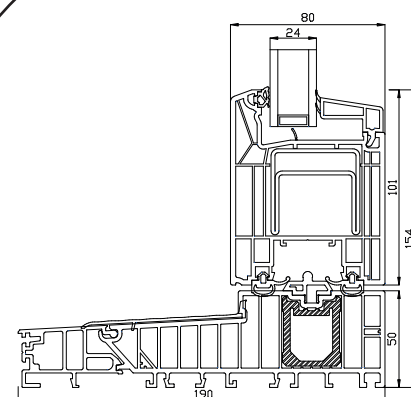
Onderdorpel
