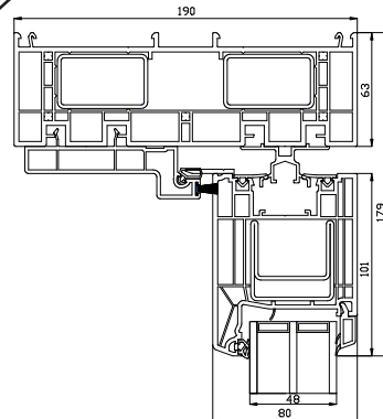
Bovendorpel
