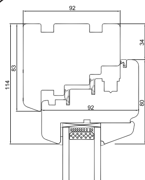
Bovendorpel
