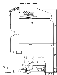
Aluminium onderdorpel
