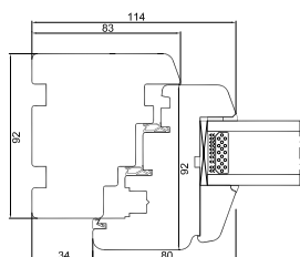
Zijstijl
