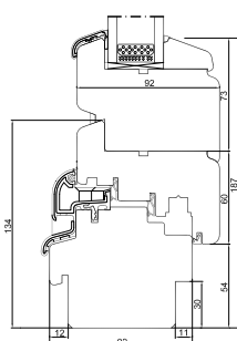
Onderdorpel hout
