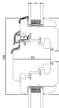
Tussendorpel
