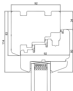
Bovendorpel
