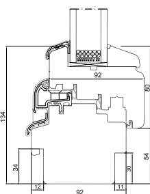
Onderdorpel
