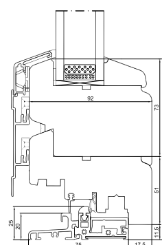
Aluminium onderdorpel
