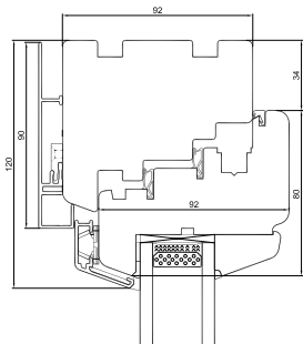
Bovendorpel
