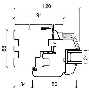
Zijstijl
