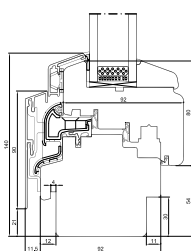
Onderdorpel
