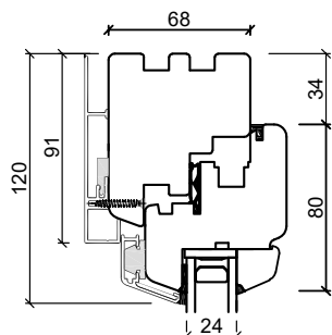
Bovendorpel
