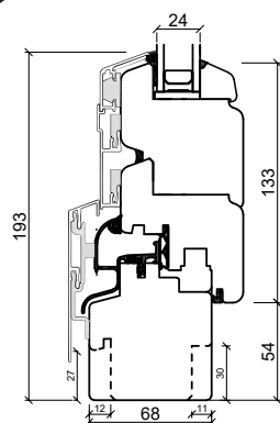
Onderdorpel hout
