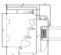
Zijstijl
