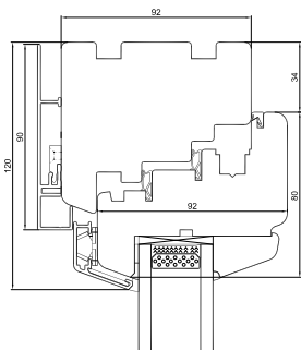
Bovendorpel
