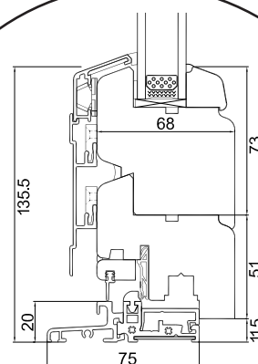
Aluminium onderdorpel
